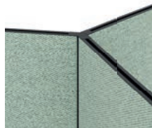
Connessione a 2/3 vie a 120° 120° 2- 3-way connection Connexion à 2/3 voies 120°
