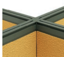
Connessione 4 vie a 90° 90° 4-way connection Connexion à 4 voies 90°
