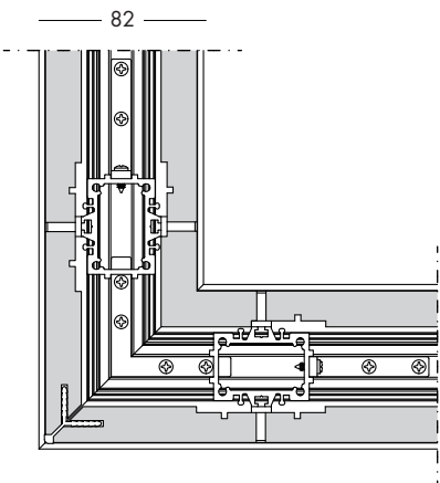
Cieco Wood partition wall Vollelementen Panneau pleine Modulo ciego
