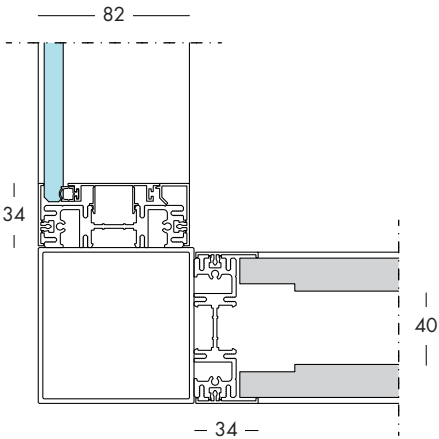
Connezione cieco e vetro offset Connection between wood panel and offset glazed Verbindung zwischen Paneele und Einzelnes Seitenglasswand Connection panneaux pleines et verre simple décentré Conexión entre los paneles y cristal singulo des centrado
