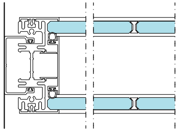
Partenza a muro per doppio vetro Wall post for double glazed Anfangsprofil für doppelverglasung Profil départ du mur avec verre double Perfil de salida para la partición con cristal doble
