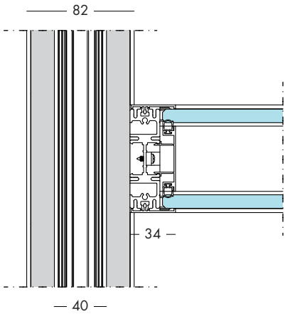
Doppio vetro su cieco 3-ways connection between wood panel and double glazed 3-Wege Verbindung zwischen Voll Panel und Doppelverglasung Connection à 3 voies panneau plein et verre double Conexión 3 vías entre el panel y cristal doble
