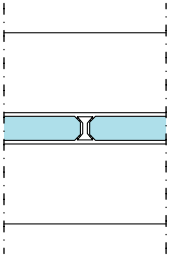
Giunto di connessione in policarbonato Polycarbonate joint Polykarbonateckverbindung Jonction en polycarbonate Perfiles de conexion en policarbonato
