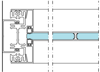
Partenza a muro per monovetro Wall post for single center glazed Anfangsprofil für zentral Glastrennwand Profil départ du mur avec verre simple centré Perfil de salida para la partición con cristal singulo centrado
