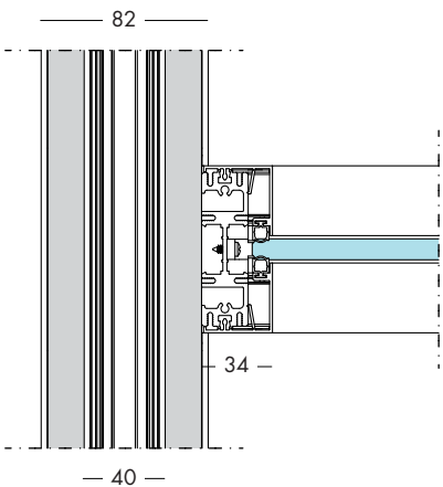
Monovetro su cieco 3-ways connection between wood panel and single center glazed 3-Wege Verbindung zwischen Voll Panel und Zentral Einfachverglasung Connection à 3 voies panneau plein et verre simple centré Conexión 3 vías completo del panel y cristal singulo centrado
