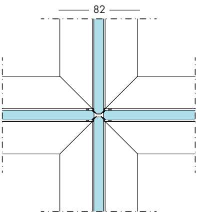
Monovetro Single glazed Zentral Einfachverglasung Verre simple centré Cristal singulo centrado
