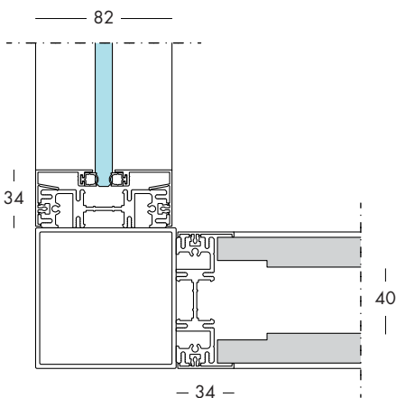
Connezione cieco e monovetro Connection between wood panel and single center glazed Verbindung zwischen Paneele und zentral Einfachverglasung Connection panneaux pleines et verre simple centré Conexión entre los paneles y cristal singulo centrado
