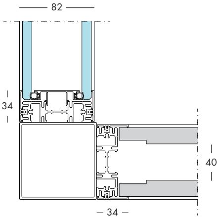
Connezione cieco e vetro doppio Connection between wood partition wall and double glazed Verbindung zwischen Paneele und Doppelverglasung Connection panneaux pleines et verre double Conexión entre los paneles y cristal doble
