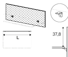
4. vasca cablaggio ispezionabile
