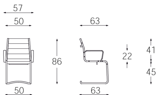
Base slitta c/braccioli - Visitatore Imbottitura poliuretano espanso
