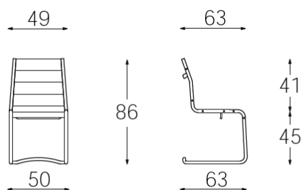
Base slitta - Visitatore Imbottitura poliuretano espanso
